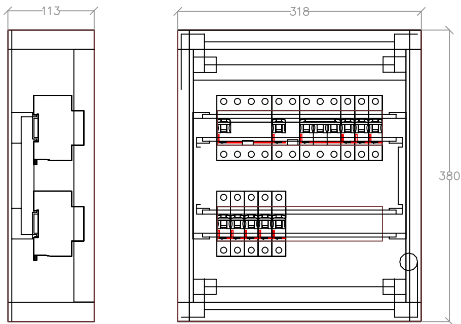
TABLICA ROZDZIELCZA TR
